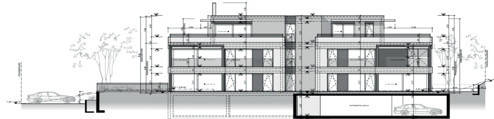
FASSADE SÜD
