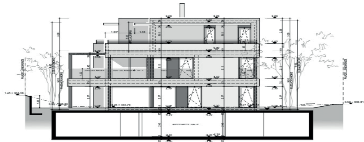
FASSADE OST
